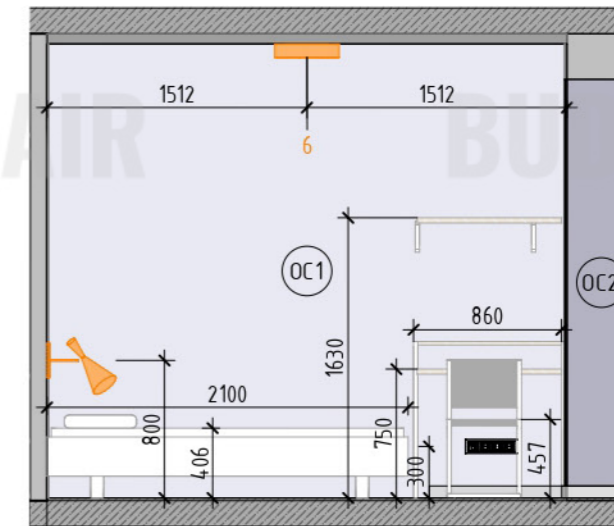
Развертка 5.2 (1 : 40)
