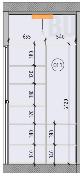
Развертка 2.2 (1:30)
