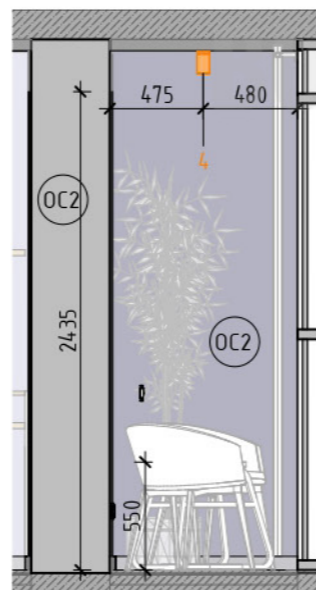
Развертка 6.2 (1 : 35)
