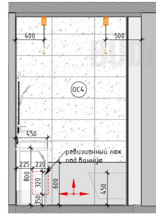
Развертка 3.4 (1:30)
