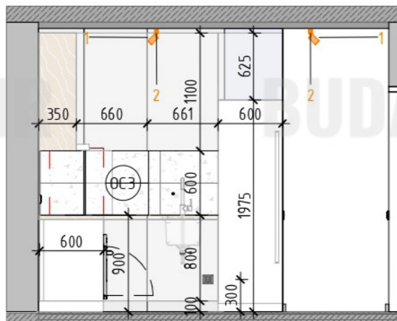
Развертка 4.1 (1: 45)
