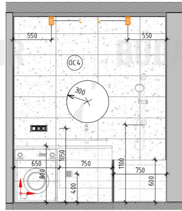
Развертка 3.3 (1:30)
