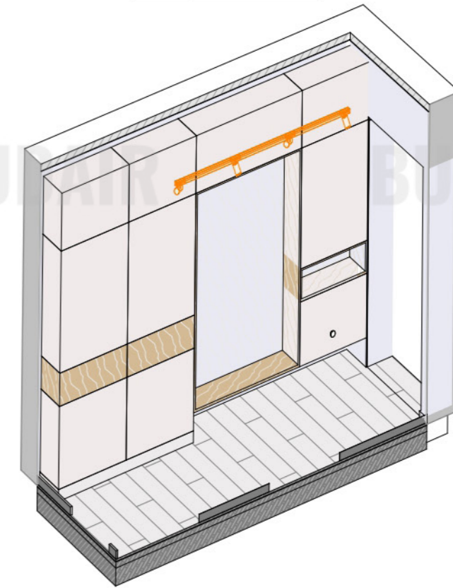
Развертка 1.4 (1: 35)
