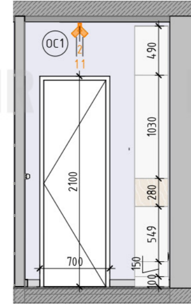
Развертка 1.4 (1: 35)
