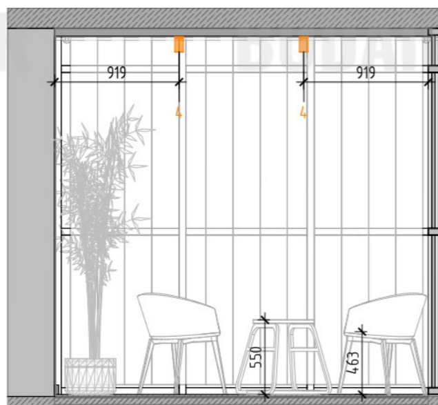
Развертка 6.1 (1 : 35)
