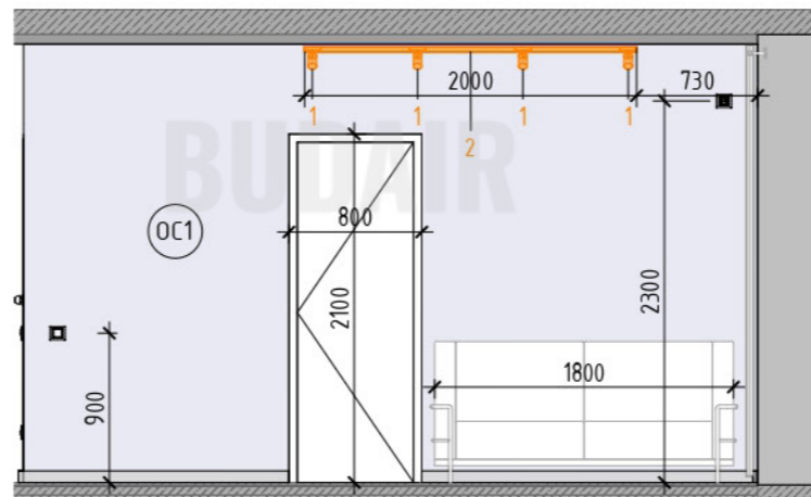
Развертка 4.2 (1: 45)
