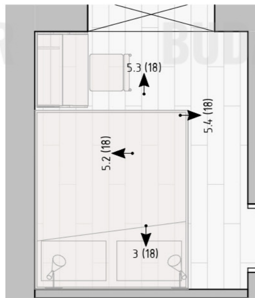
Помещение 5, Спальня (1 : 40)
