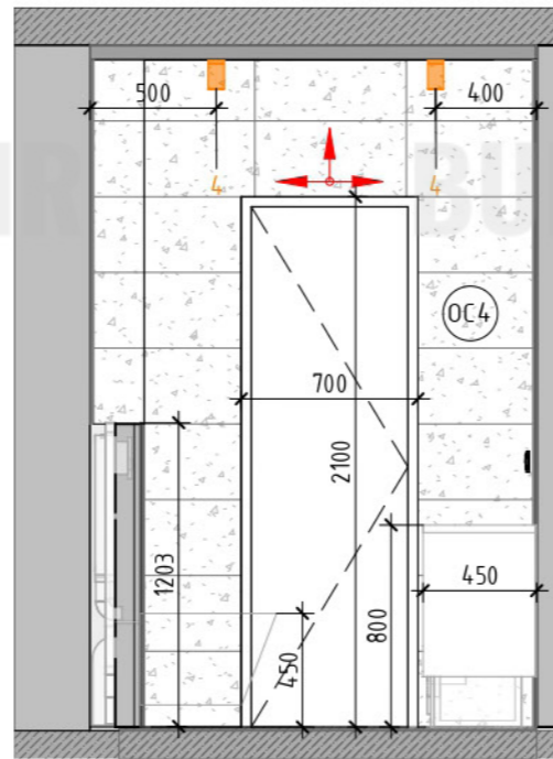
Развертка 3.2 (1:30)
