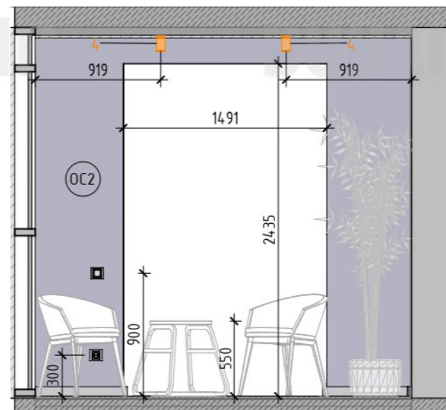
Развертка 6.3 (1 : 35)
