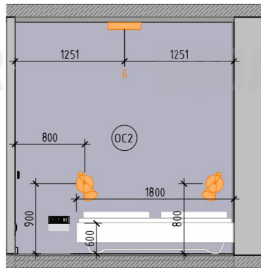
Развертка 5.1 (1 : 40)
