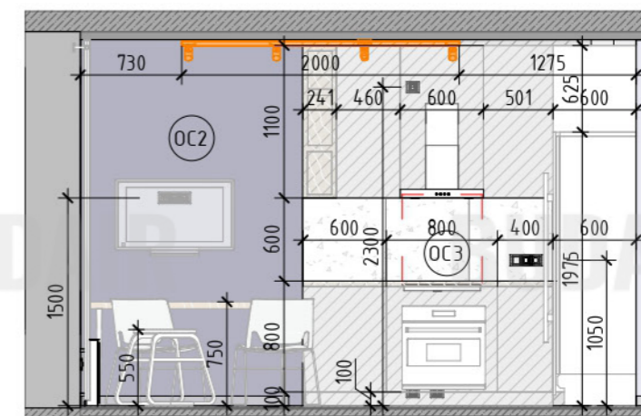
Развертка 4.4 (1: 45)
