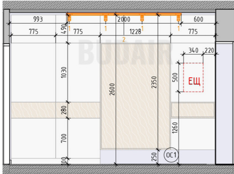
Развертка 1.1 (1: 35)
