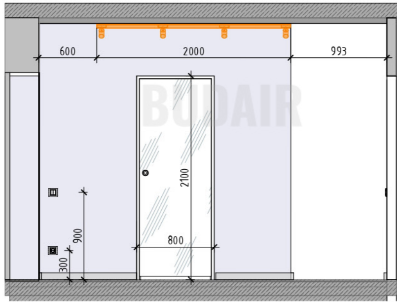
Развертка 1.3 (1: 35)
