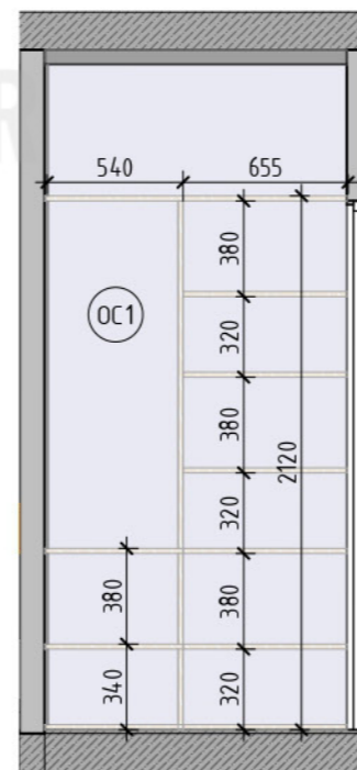
Развертка 2.4 (1:30)
