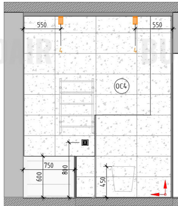
Развертка 3.1 (1:30)
