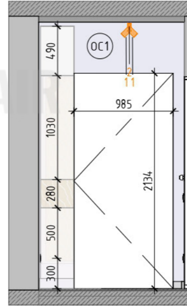
Развертка 1.2 (1: 35)
