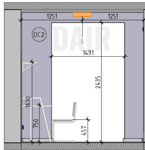
Развертка 5.3 (1 : 40)
