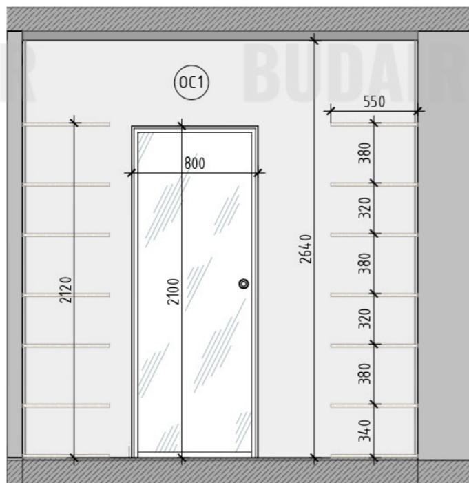
Развертка 2.1 (1:30)
