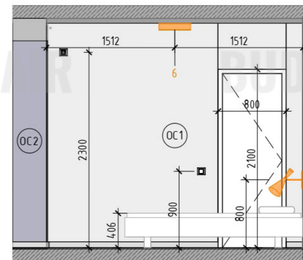
Развертка 5.4 (1 : 40)
