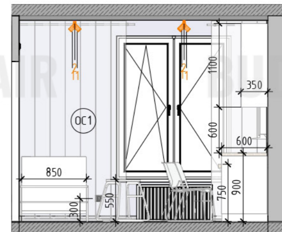
Развертка 4.3 (1: 45)
