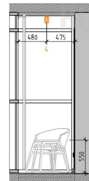
Развертка 6.4 (1 : 35)
