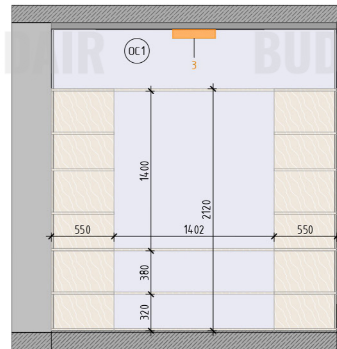
Развертка 2.3 (1:30)
